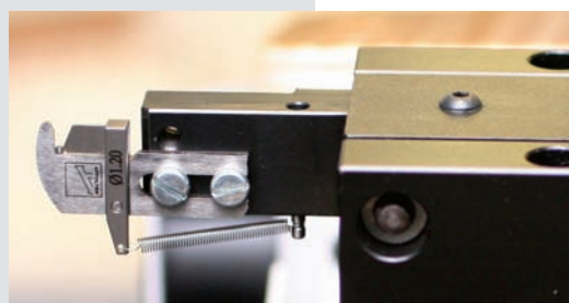
Brucelles de chargement type AF20
