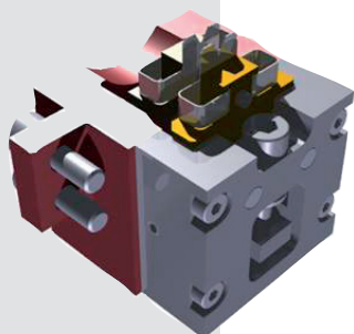
Tête réglable avec centrage en «v»
